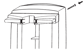
ポールステー(ポール用取付器具)取付方法
